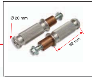
RP56 € 32,50 Coppia poggia piedi corti short footpegs (pair) colori: nero, ergal colours: black, ergal
