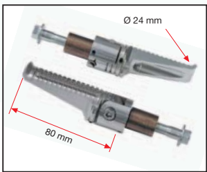
KSN01 € 88,00 coppia pedane poggia piedi Tipo 3 type 3 footpegs (pair)
