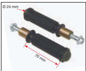
RP49 € 48,00 Coppia poggia piedi Tipo 3.5 type 3.5 black footpegs (pair)
